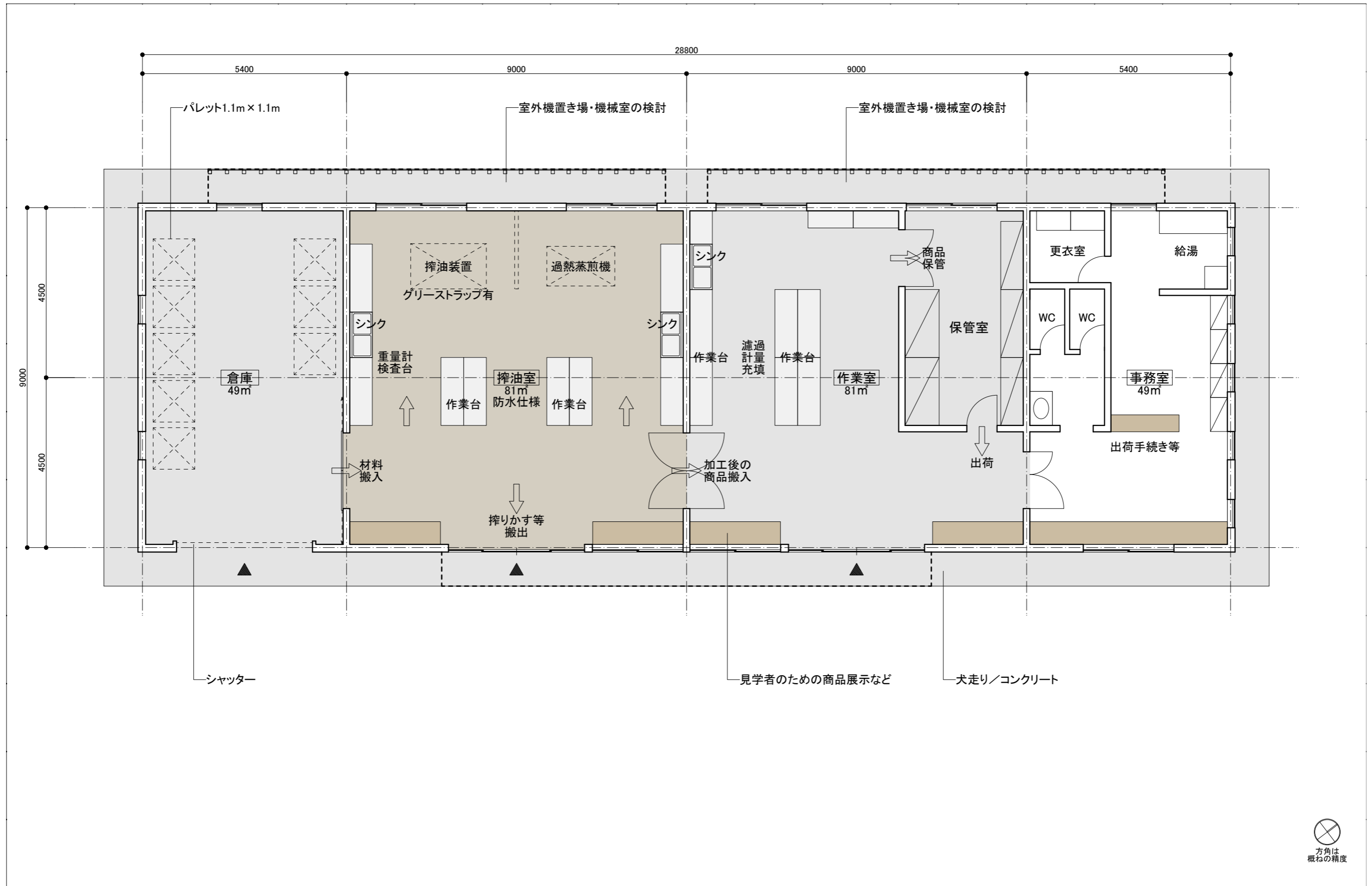
平面図
