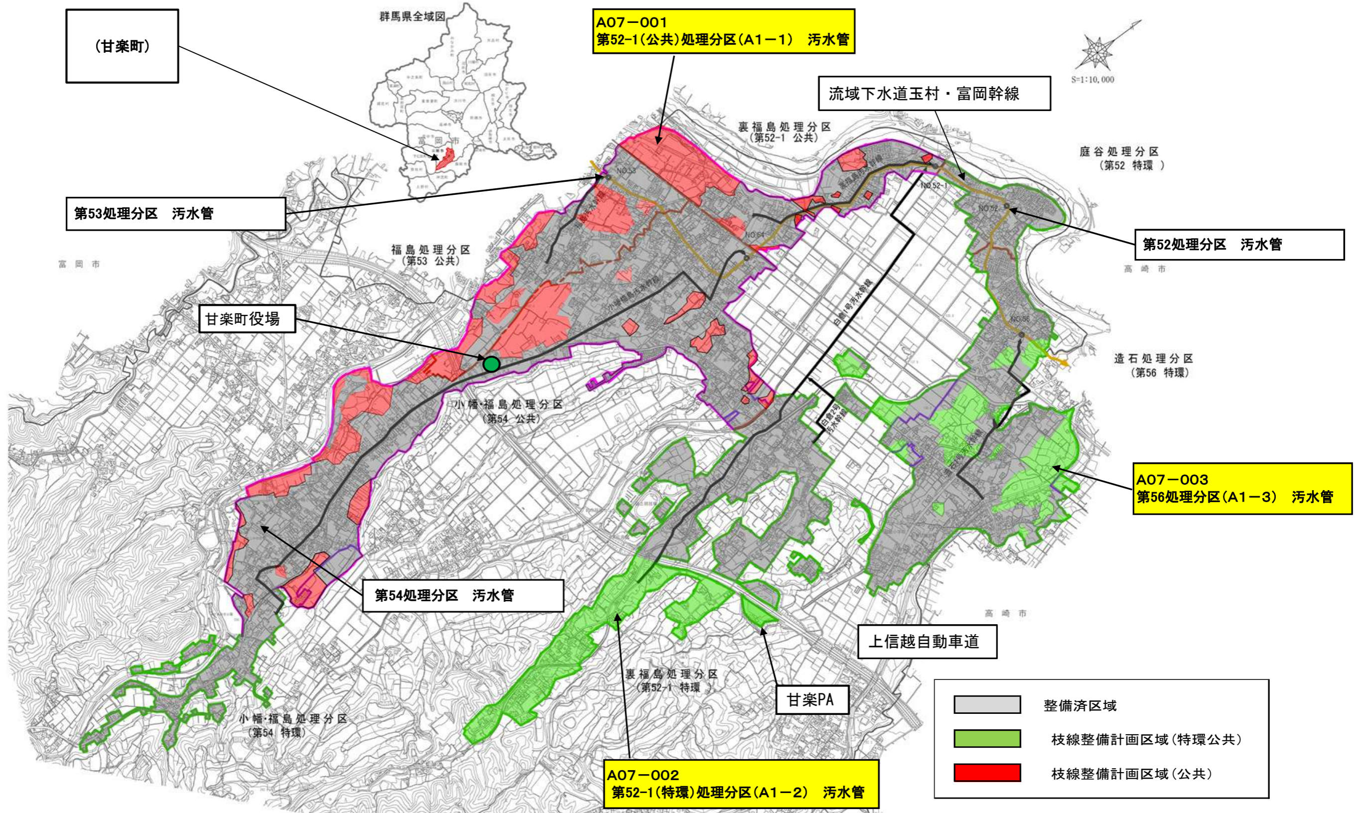
甘楽町(県央処理区)計画図
